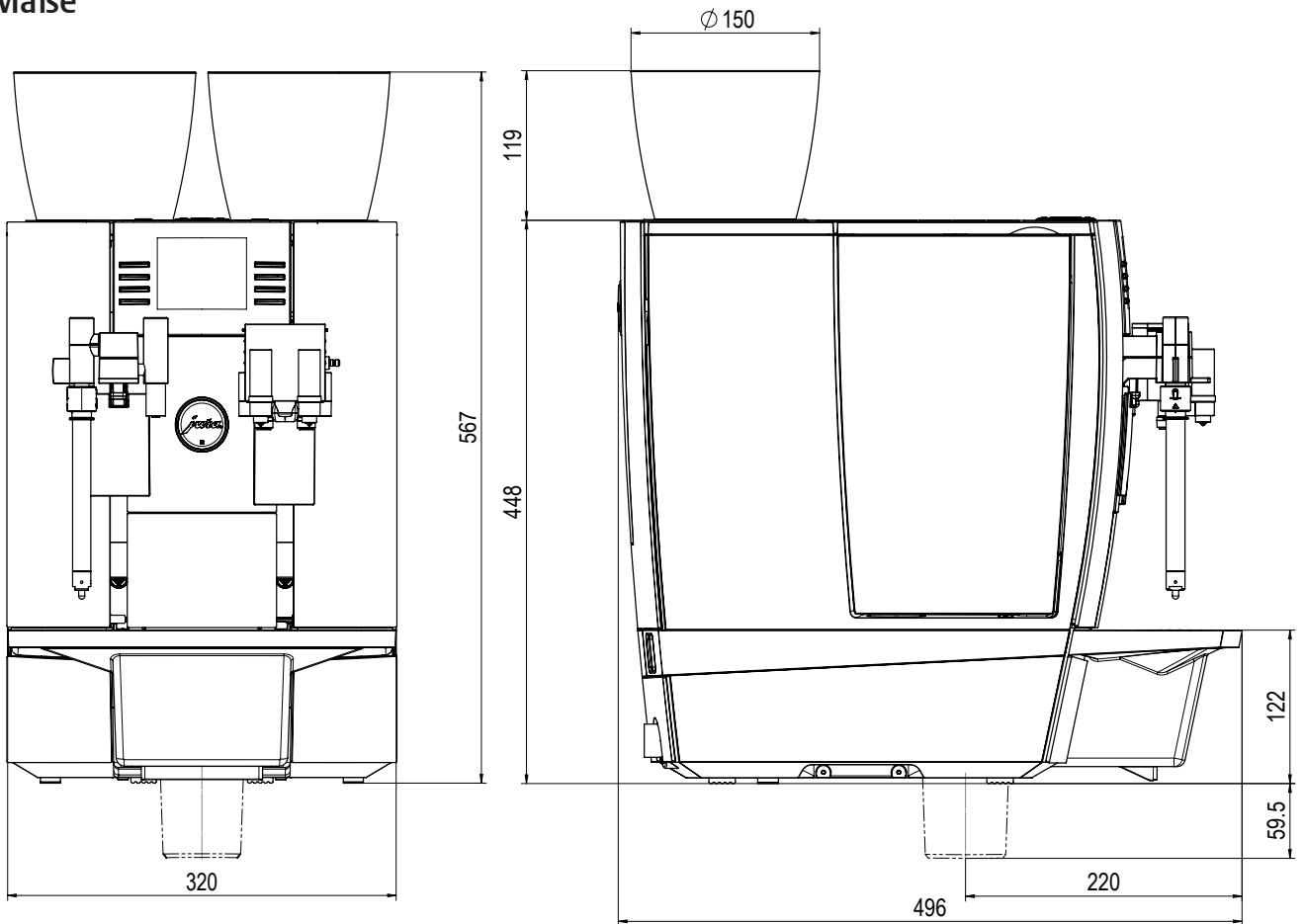
Aufriß
